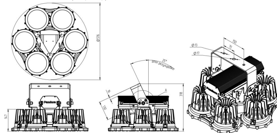
Рисунок 1. Габаритный чертеж
